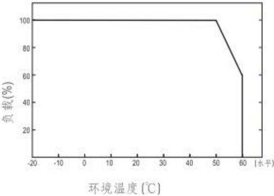
衰减曲线
