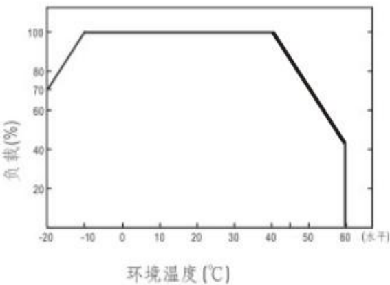
衰减曲线
