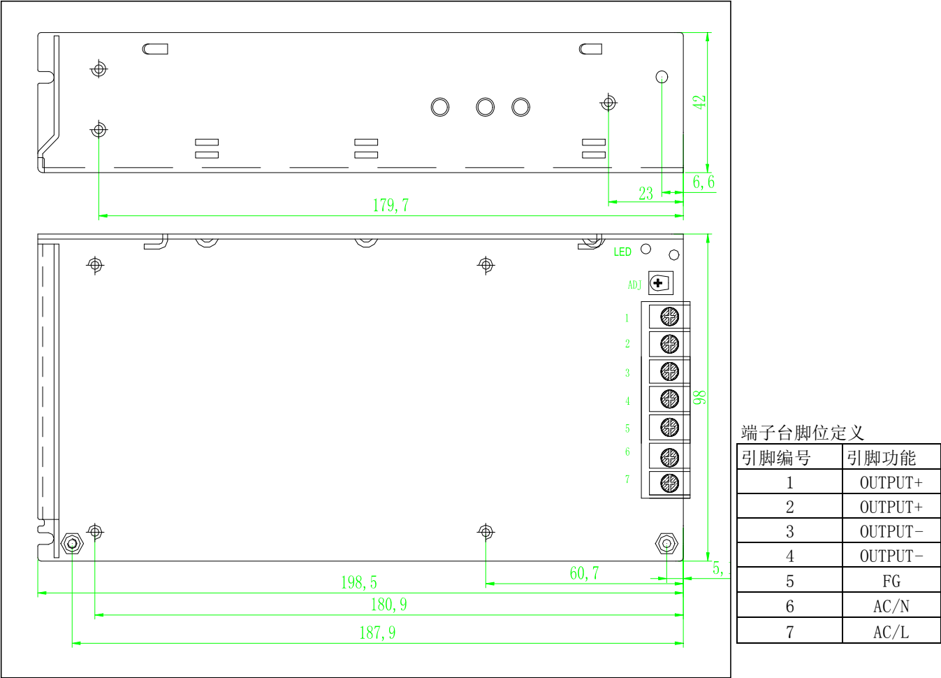
外形结构
